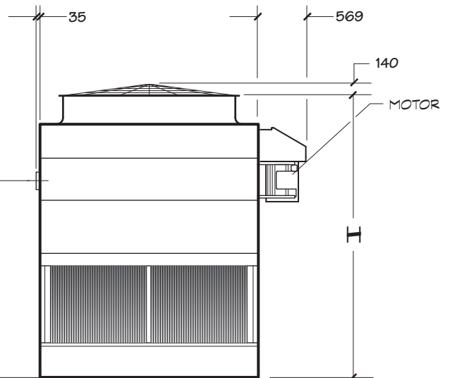
END ELEVATION
