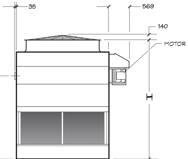
END ELEVATION
