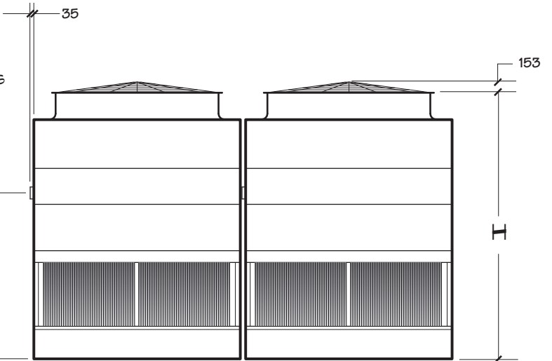
END ELEVATION
