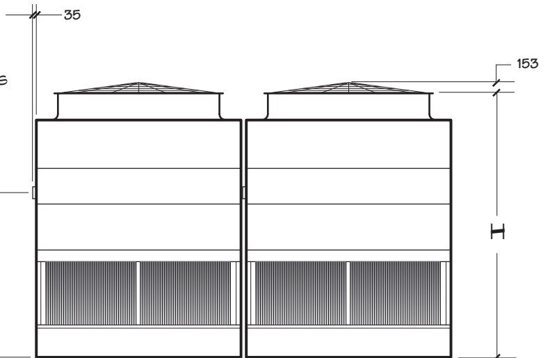
END ELEVATION
