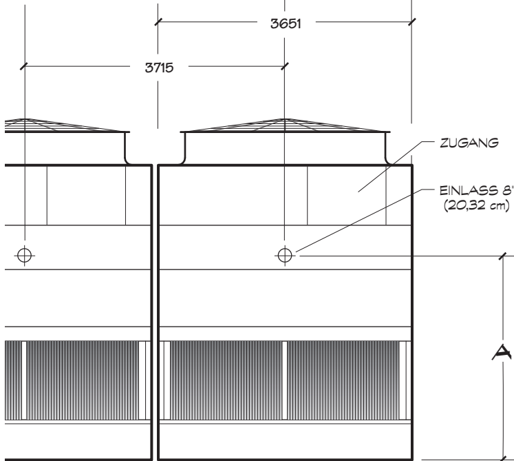
SEITENANSICHT LÄNGSSEITE
