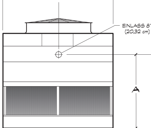
SEITENANSICHT LÄNGSSEITE
