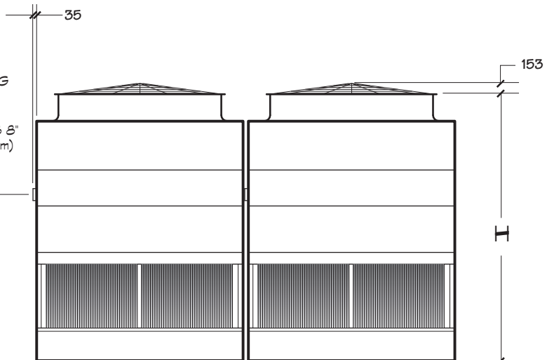
SEITENANSICHT BREITSEITE
